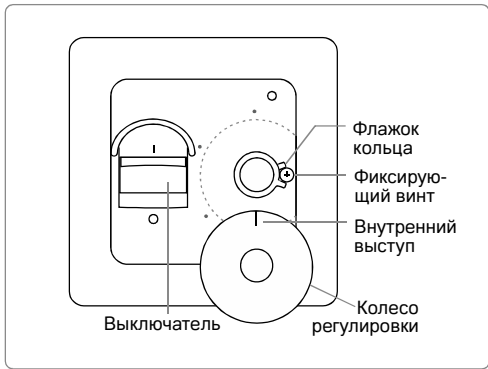
Рисунок 2. Схема терморегулятора и блокировка управления с помощью фиксирующего винта
